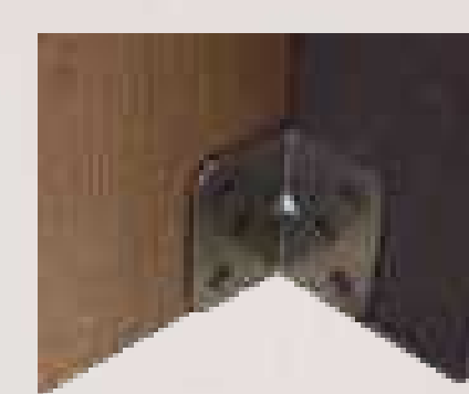
L-CLIP 50x50x1.2mm
